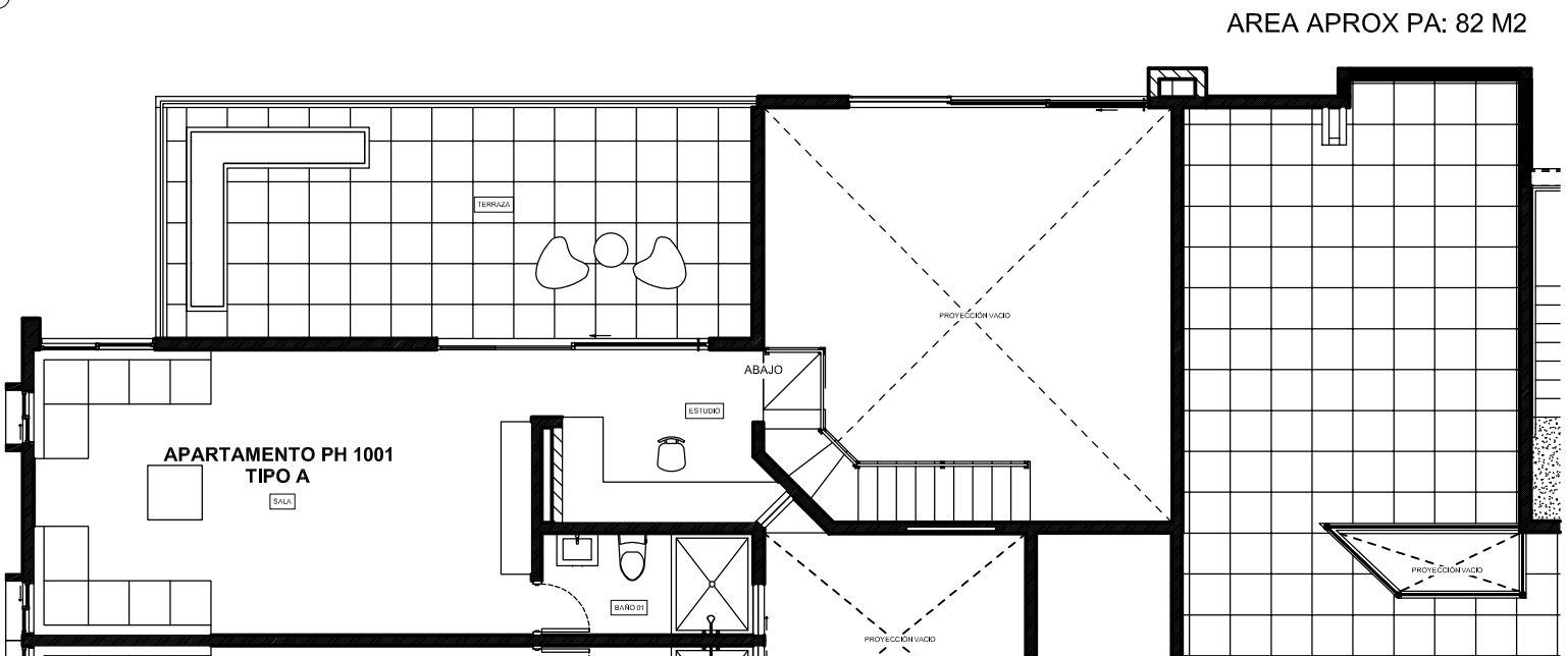
3 PLANTA GENERAL APTOS TIPO A PISO 11
